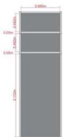
14 PAINEL DE TS MATERIAL: ADESIVO IMPRESSO APLICAÇÃO: SOBRE TS
