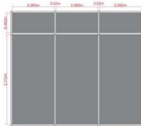
5 PAINEL DE TS MATERIAL: ADESIVO IMPRESSO APLICAÇÃO: SOBRE TS
