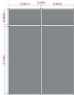
4 PAINEL DE TS MATERIAL: ADESIVO IMPRESSO APLICAÇÃO: SOBRE TS
