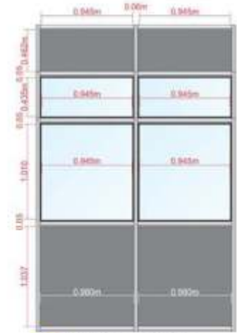
13 PAINEL DE TS/VIDRO MATERIAL: ADESIVO IMPRESSO APLICAÇÃO: SOBRE TS/VIDRO
