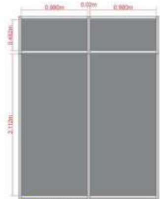
10 PAINEL DE TS MATERIAL: ADESIVO IMPRESSO APLICAÇÃO: SOBRE TS
