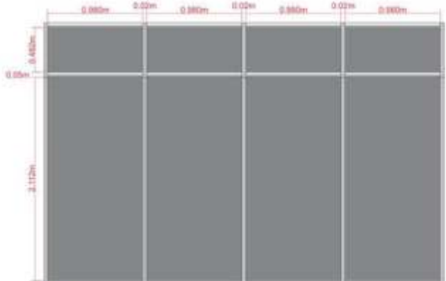
17 PAINEL DE TS MATERIAL: ADESIVO IMPRESSO APLICAÇÃO: SOBRE TS
