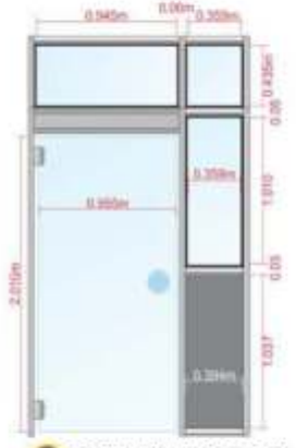
11 PORTA DE VIDRO TEMP. MATERIAL: ADESIVO IMPRESSO APLICAÇÃO: SOBRE VIDRO
