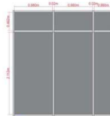
12 PAINEL DE TS MATERIAL: ADESIVO IMPRESSO APLICAÇÃO: SOBRE TS
