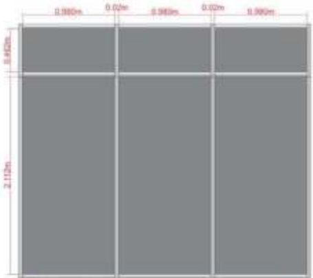
18 PAINEL DE TS MATERIAL: ADESIVO IMPRESSO APLICAÇÃO: SOBRE TS
